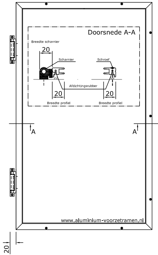
Vast met scharnieren & schroeven
