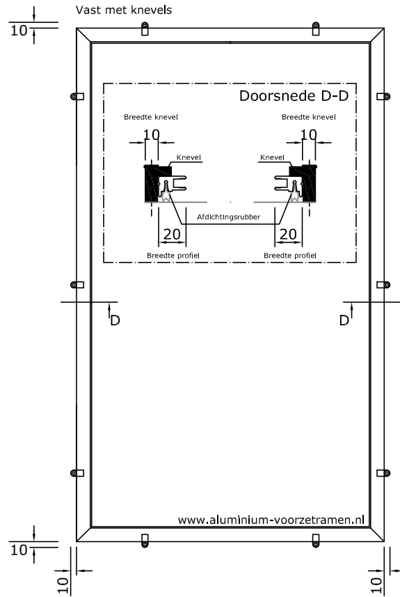
Vast met knevels
