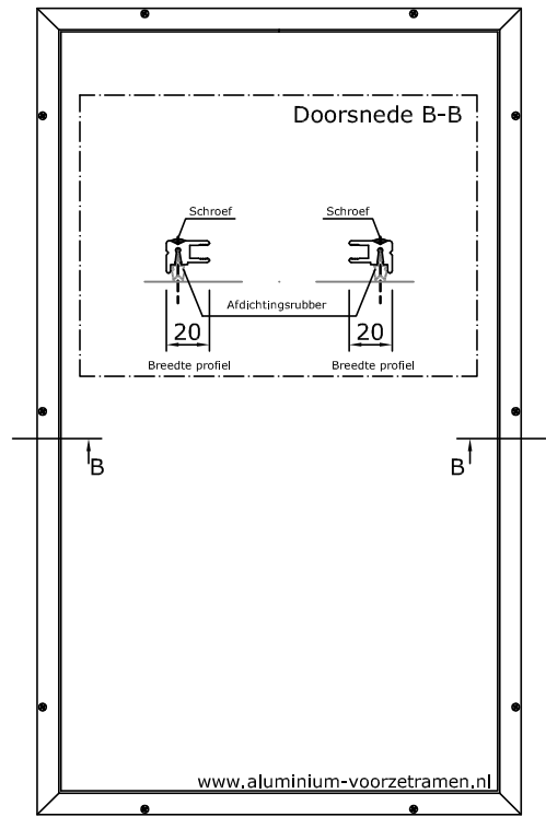
Vast met schroeven
