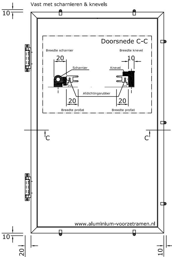
Vast met scharnieren & knevels
