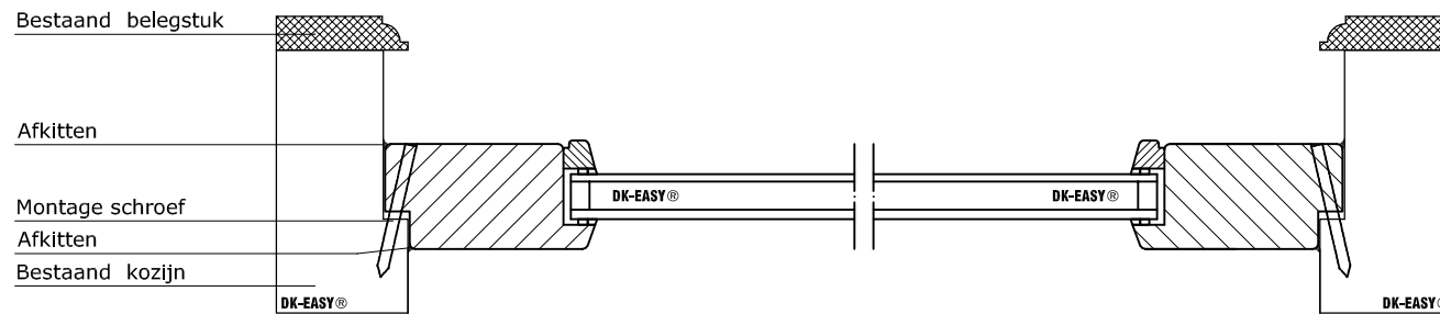
Bovenraam
