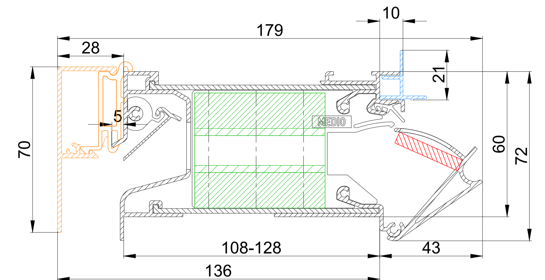
DucoTop 60 ZR Medio
