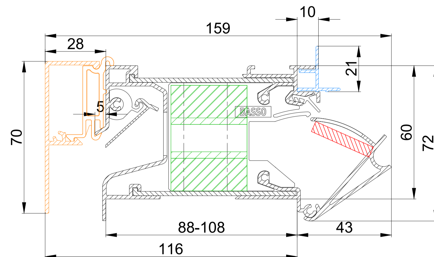
DucoTop 60 ZR Basso
