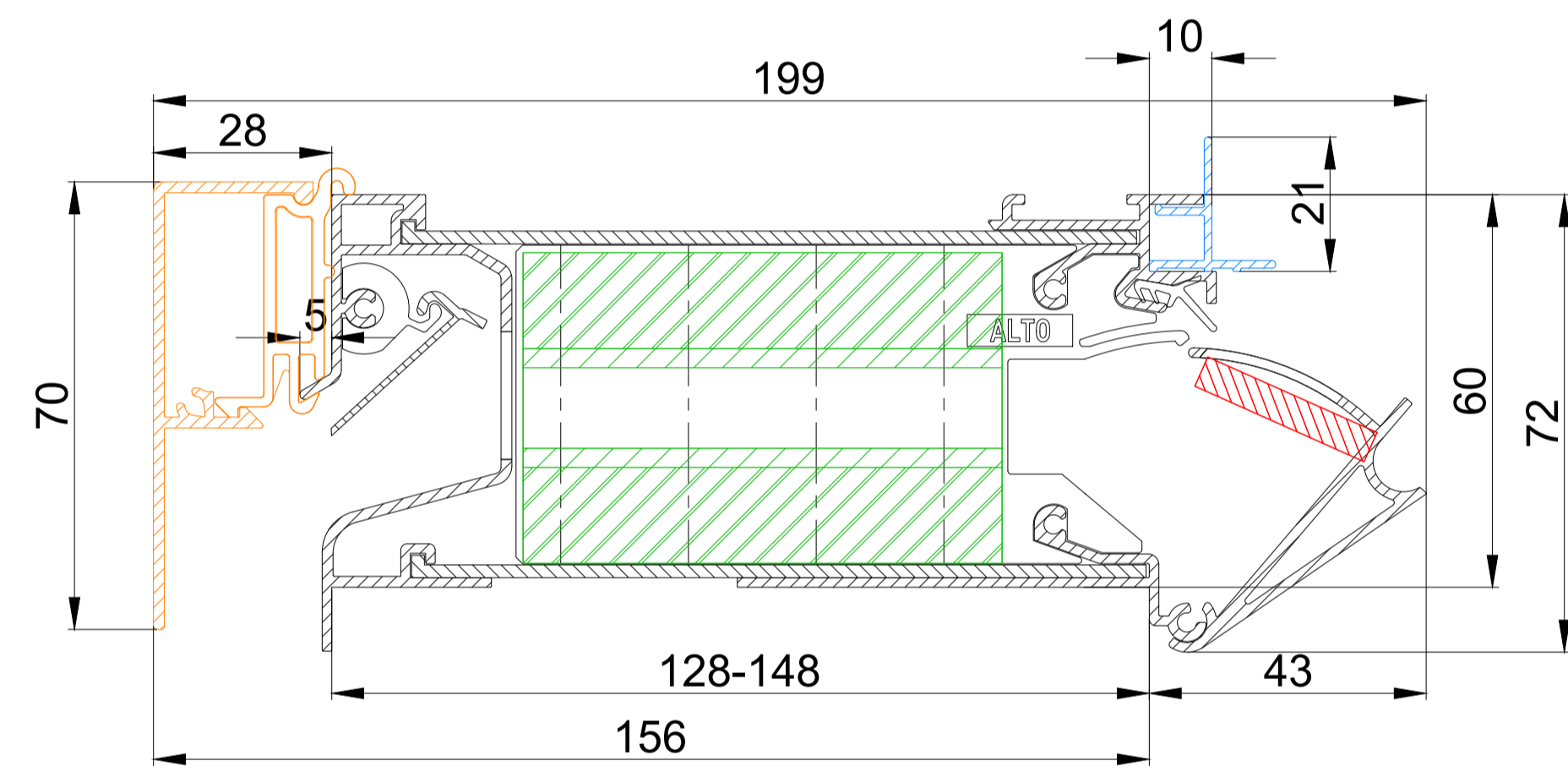
DucoTop 60 ZR Alto
