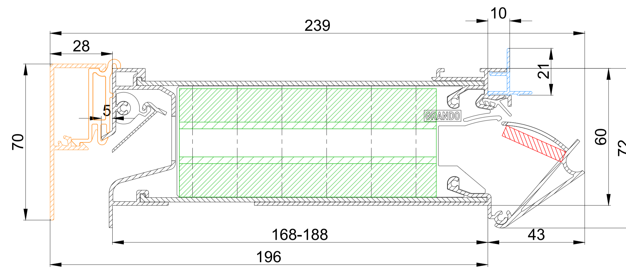
DucoTop 60 ZR Grando
