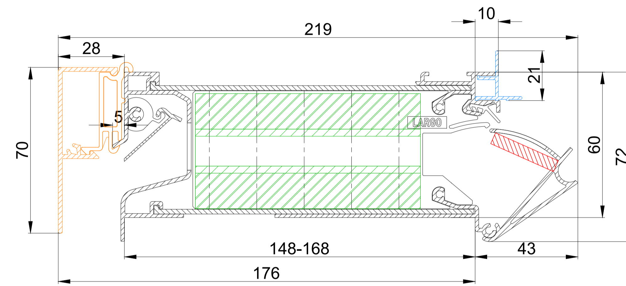
DucoTop 60 ZR Largo
