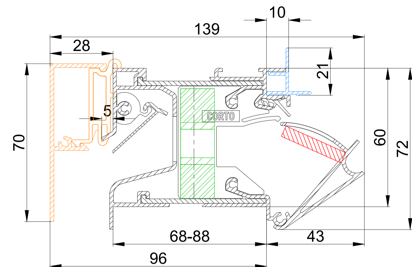
DucoTop 60 ZR Corto
